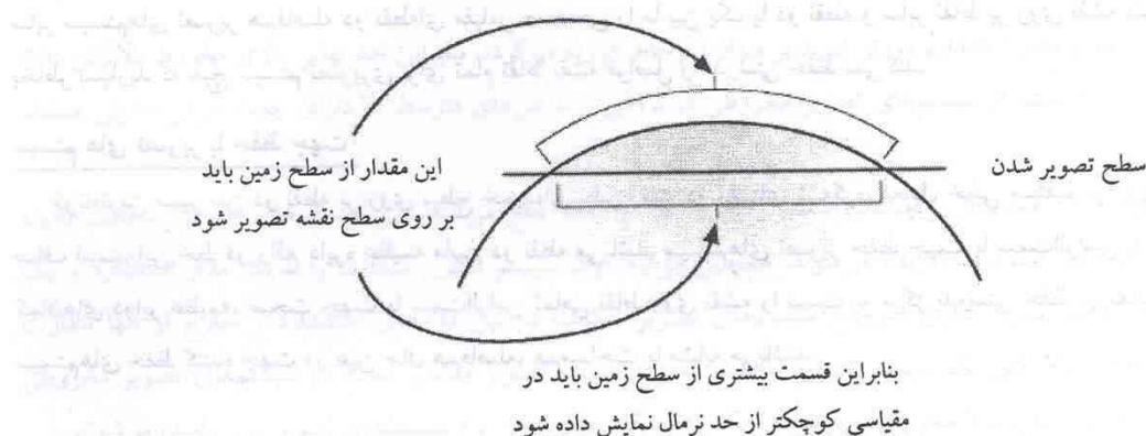
شکل (۵-۵): نحوه تصویر کردن سطح زمین بر روی سطح نقشه
