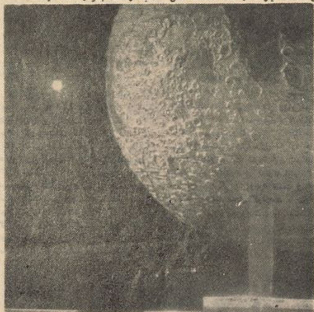
به کمک استیوت کریستال لوگراف اکادمی علمی اتحاد شوروی در فواصل میان سیاره زمین و مهابت یاقوت کشف و تشخیص گردانیده شده .
