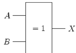
Äquivalenz
