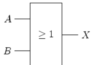
Implikation
