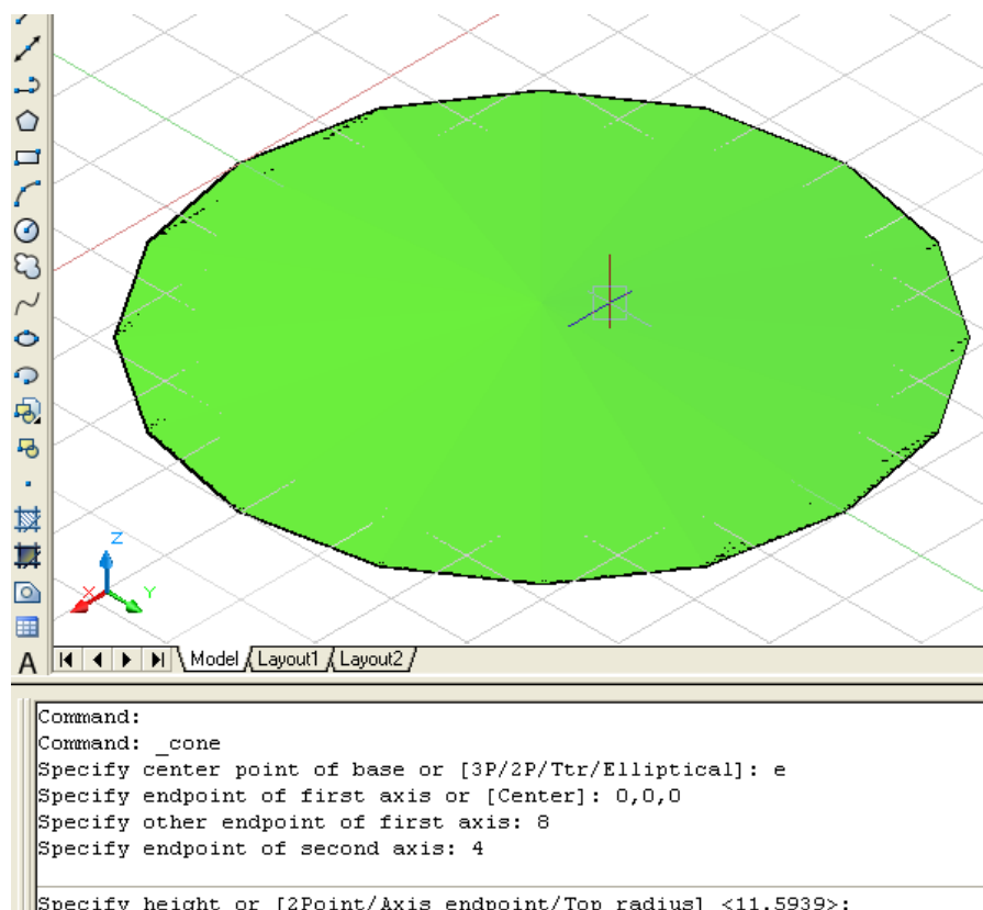
شکل د (۳۸-۱) منیو خهده مخروط (Cone) په هدايت کي دکارد شروع دمخه دلاندني سطحه رسمول د (E) له رویه اود محوروا انتخاب
