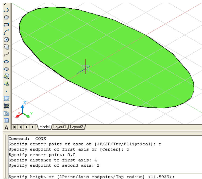
شکل د (۳۹-۱) منیو خهده مخروط (Cone) په هدايت کي دکارد شروع دمخه دلاندني سطحه رسمول د (E) له رویه او د مرکز انتخاب
