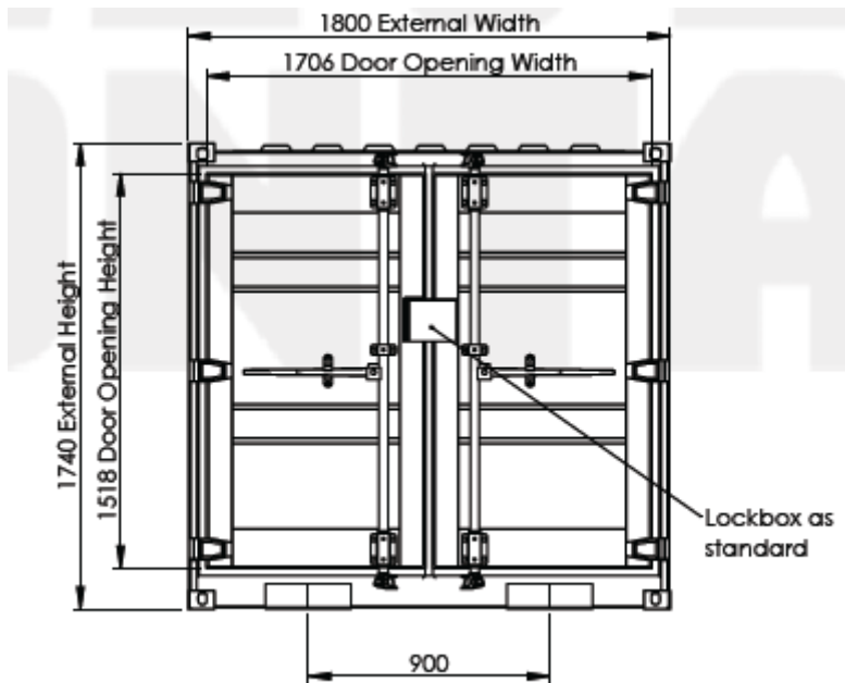
نمای دروازه کانتینر ۷ فـت مینی
