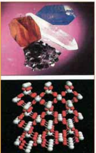
11 - 6 شکل دکوارتز بلوري جوړښت اود هغه په مالیکولونو کې د سیلیکان او اکسیجن داتومونو ځای پر ځای کیدل ښیي.
