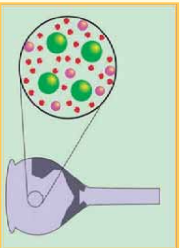
(1-2) شکل د خوړو د مالګې محلول ، د ایونونو او اوبو د مالیکولونو خپریدل د محلول په ټولو برخو کې
