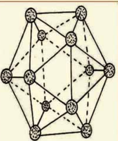
(1-1) شکل د بورون د الوتروپي بلوري جوړښت چې 12 اتومي انگز وېر بنسټ جوړ شوی دی
