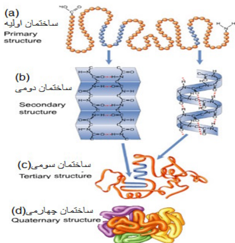
شکل 4: ساختمان پروتئین.
