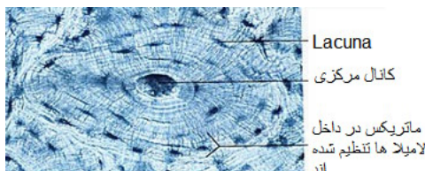
شکل 24: نسج استخوانی.
