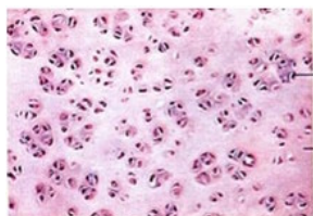
شکل 21: غضروف شفاف.
