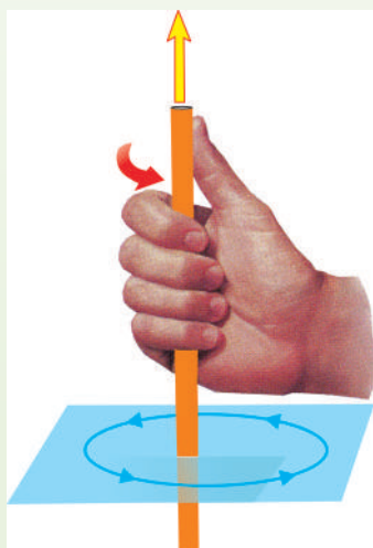
(8-9) شکل: د B د ټاکلو لپاره د ښي لاس
