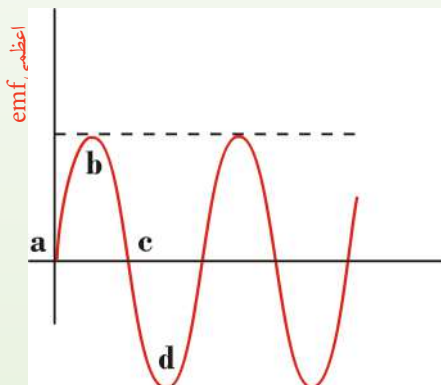
(9-20) شکل: په څرخېدونکي حلقه کې القا شوي تغیر د
