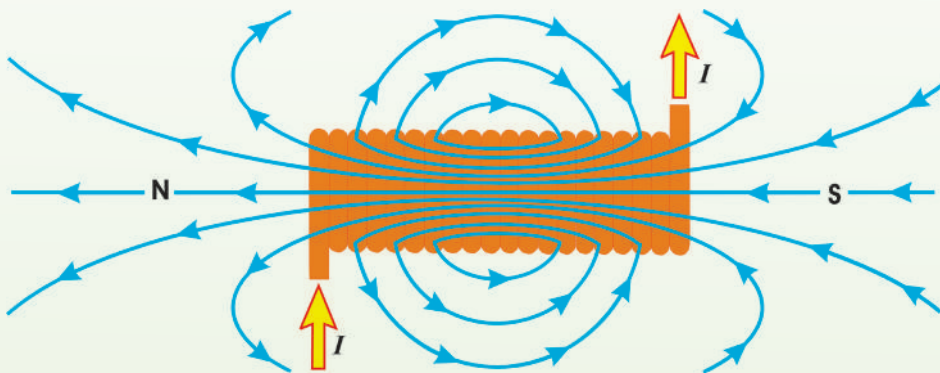
(8-12) شکل: د سولینویډ په دننه کې ساحه غښتلي او منظمه ده.
