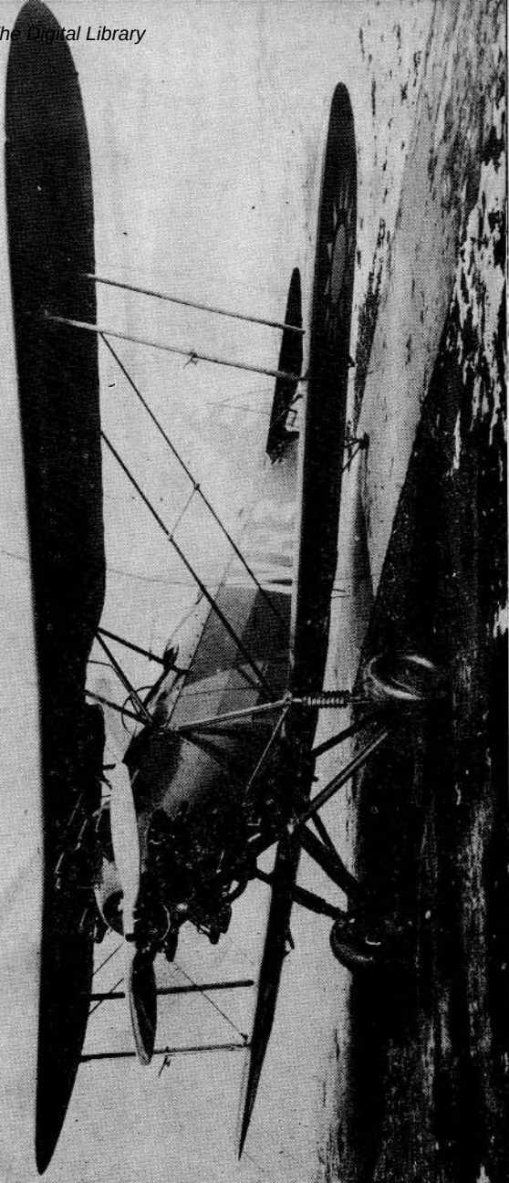
ازکار روائی های سال ۱۳۱۶ وزارت حربیه : نمونه طیارات تعلیمی رقم « بردا ۲۵ » ایتالوی که جدیداً خریداری شده Type des nouveaux avions d'enseignement achetés par le ministère afghan de la guerre
