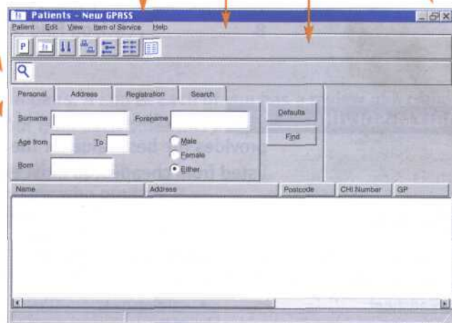
Fig 3 GPSS
